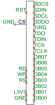
5" SSD1963 Display
